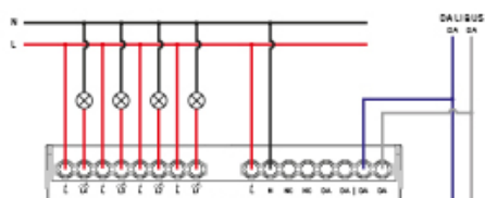
SCHÉMA DALI
