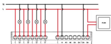
SCHÉMA PAR LA PHASE / PD
