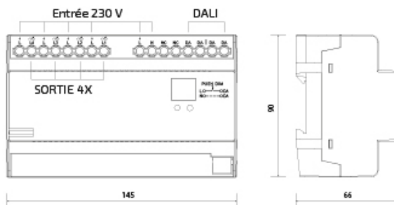
SCHÉMA DALI
